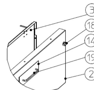
DETAIL1 Maßstab 1:10
