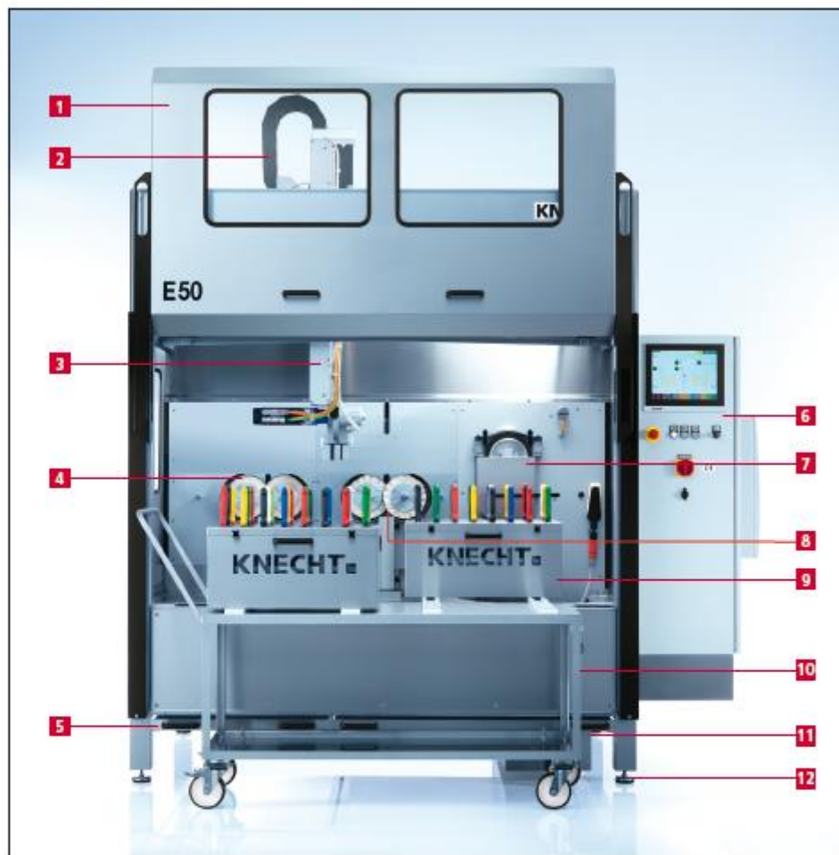
Bild 3-2 Gesamtansicht Schleifmaschine
