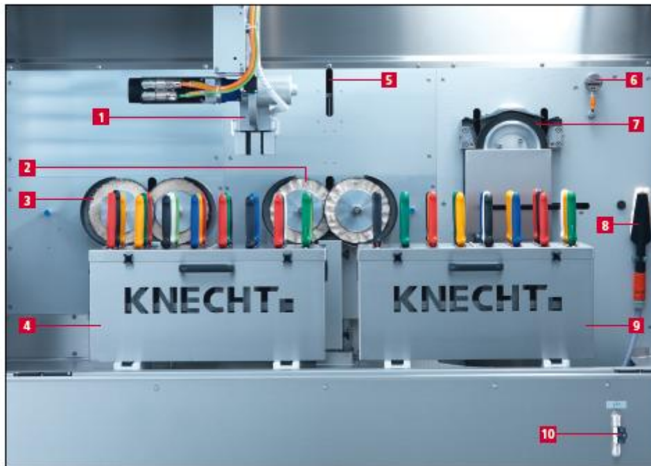
Bild 3-3 Innenraum
