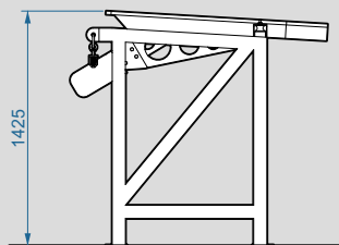
ALZADO ALIMENTADOR VIBRANTE xxx
