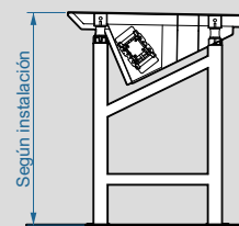
ALZADO ALIMENTADOR VIBRANTE 590
