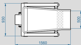
PLANTA ALIMENTADOR VIBRANTE xxx
