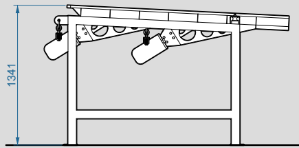
ALZADO ALIMENTADOR VIBRANTE xxx
