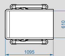
PLANTA ALIMENTADOR VIBRANTE 590
